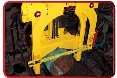
通过轨道切割运动快速切割管道, 锯片寿命大大延长
